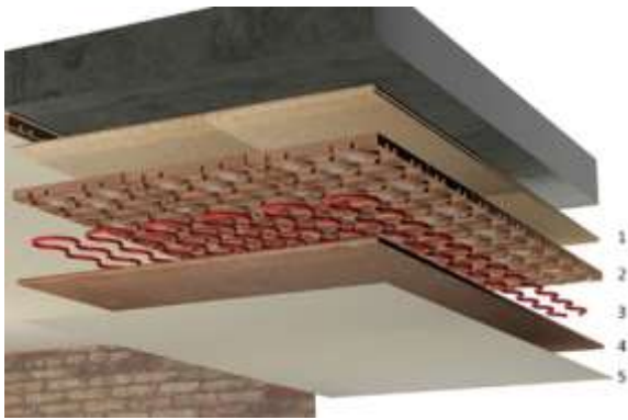
Bild 5: Konstruktionsaufbau
