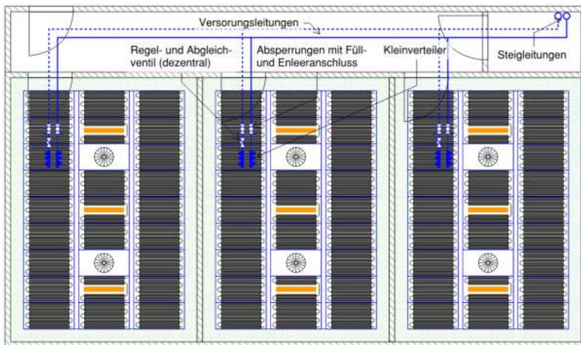
Bild 13: Dezentrale Anordnung der Regel- und Reguliereinrichtungen mit Kleinverteilern
