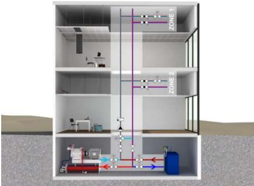
Bild 10: 2-Leitersystem
