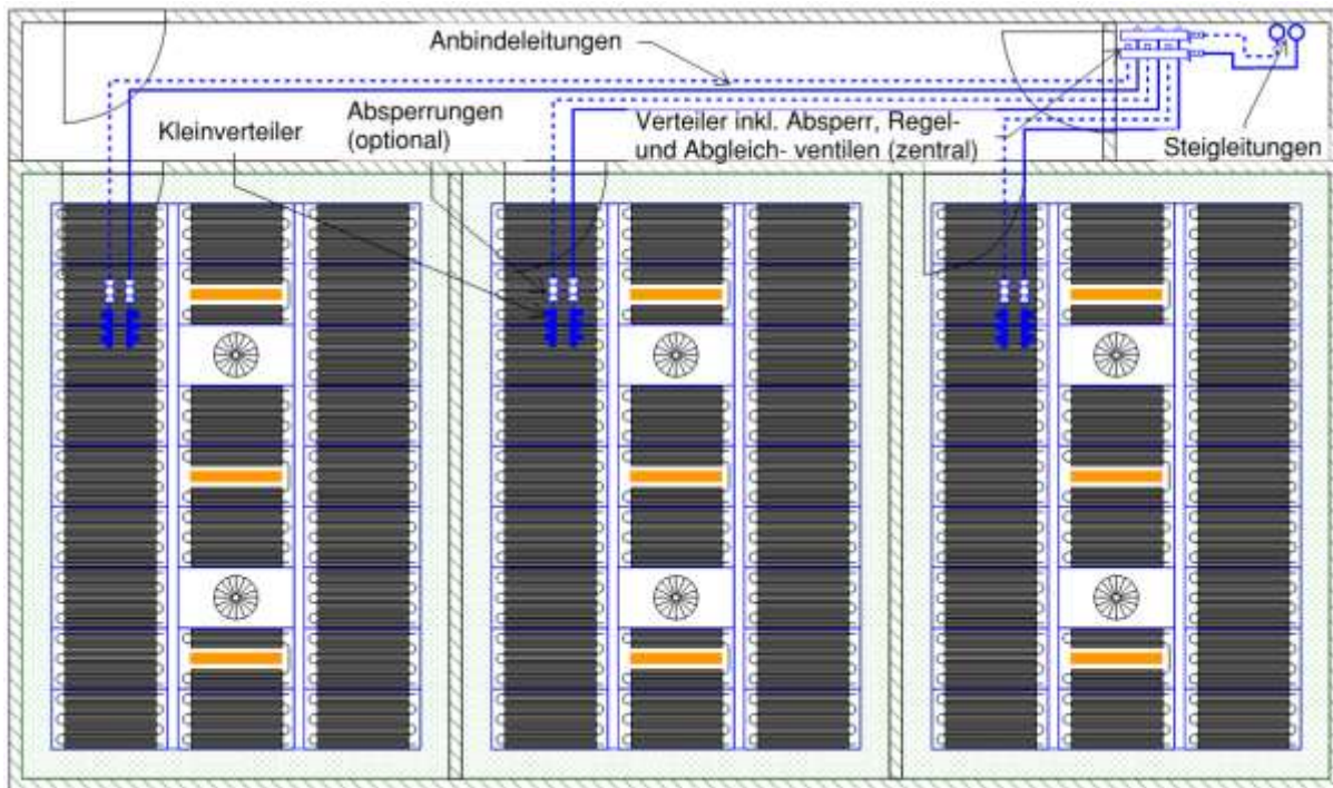
Bild 12: Zentrale Anordnung der Regel- und Reguliereinrichtungen mit Kleinverteilern
